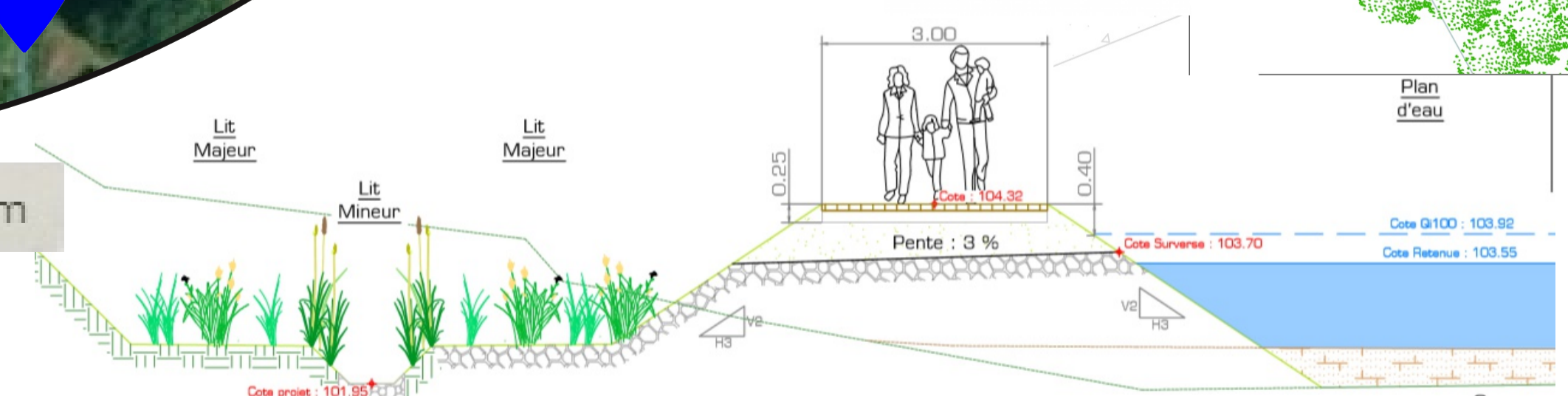
Profil de la surverse Echelle : 1/775
